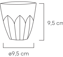
Bicchieri Ankon realizzati in materiale SAN Balance®. Dimensioni: ø9,5x9,5 h cm
